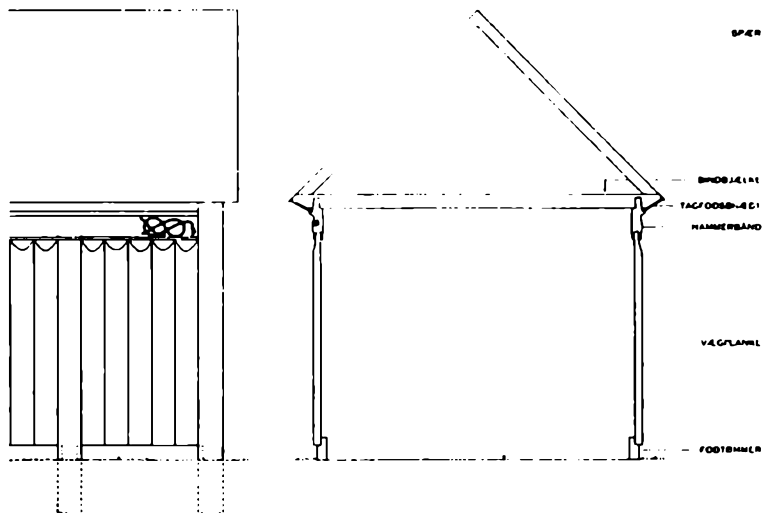
(fig. 9) Opstalt og snit til anskueliggørelse af konstruktionsprincipper m. v. Tegningen må ikke opfattes som et forsøg på rekonstruktion af Høring trækirke.
