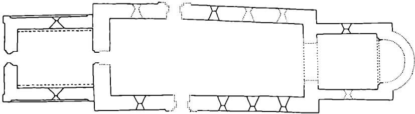
Toreby Kirke før 1300, inden tårnets forhøjelse og tårnspindeltrappens indbygning i tårnets nordvestlige hjørne, plan 1:400.
