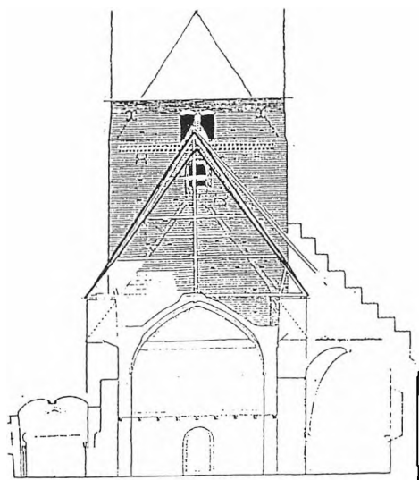
Måleblad af tårnets østside og snit i kirkens hovedskib og sideskibe, 1:400. Under det nuværende tag ses tydeligt tagsporet efter den romanske kirkes tag før hovedskibets forhøjelse i det 15. århundrede. Det gotiske tagværk fra 1500-1505 er optrukket med kraftig streg og under dette er med tilsvarende streg markeret, hvor det genbrugte romanske tagværk stod indtil det blev kasseret, da hovedskibet fik hvælv og nyt tagværk.
