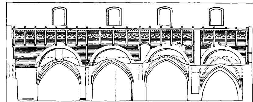
Hovedskibets sydside (søndre sideskib bortskåret), 1:200. Den romanske kirkes fire vinduer giver sig alle til kende og af mandsdørens murede fremspring anes den vestre kant. Bemærk de store rundbuede udhugninger i muren, nu delvis tilmurede, men oprindeligt, før der blev bygget hvælv i søndre sideskib, åbne mod hovedskibet. Den lave spidsbue til det ældre, søndre kapel ses tydeligt.
