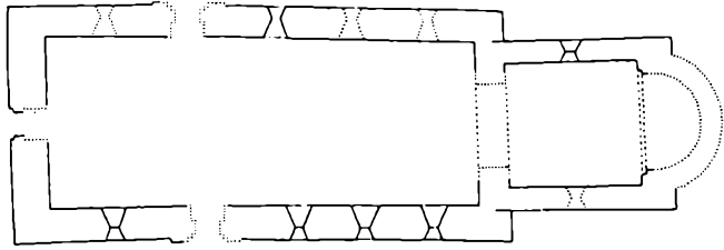
Toreby Kirke ca. 1250, plan 1:400. Det meget store kirkeskib har mandsdør i syd, kvindedør i nord og vestportal, som sjældent forekommer ved landsbykirker. Bemærk, at der ikke er symmetri i døres og vinduers anbringelse i syd- og nordside.
