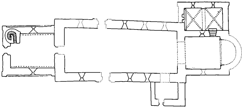
Toreby Kirke efter tilbygning af sakristi på korets nordside omkring år 1300 og kapel på sydsiden, plan 1:400. Bemærk tårmspindeltrappen.
