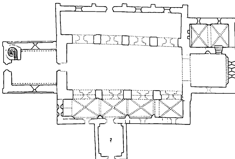
Toreby Kirke i sidste halvdel af det 15. århundrede, plan 1:400. Hovedskibet er blevet forhøjet omkring århundredets midte og siden er nordre sideskib bygget, men hvælvslagning er ikke udført i koret (ca. 1500) og i hovedskibet (1500-1505). Nordre sideskibs hvælv indbygges omkring Reformationen. Våbenhuset er antagelig bygget før 1500, men dateringen af denne bygning er højst usikker, da murværket er stærkt fornyet overalt.
