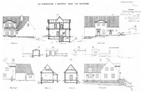
Arkitekt Plums tegninger fra 1923 til Vilhelm Arnesens nye villa på Skansørevej. Helsingør Kommunes byggesagsarkiv.
