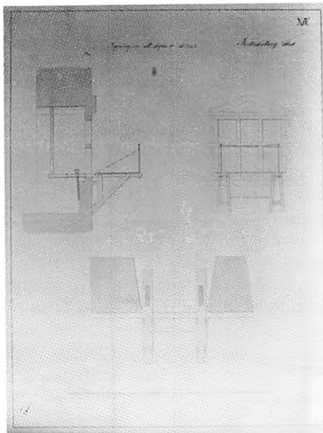
Kun få af Zwingmanns tegninger er bevaret. En af disse er "Tegning af et flytbart Stillads - Frederiksborg Slot" dateret 1860 og med signaturen CZ. (Frederiksborgmuseet)
