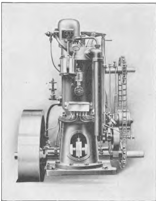
4 Takts Petroleums- og Raaoile-Motor fra Motorfabriken „Meteor“.
