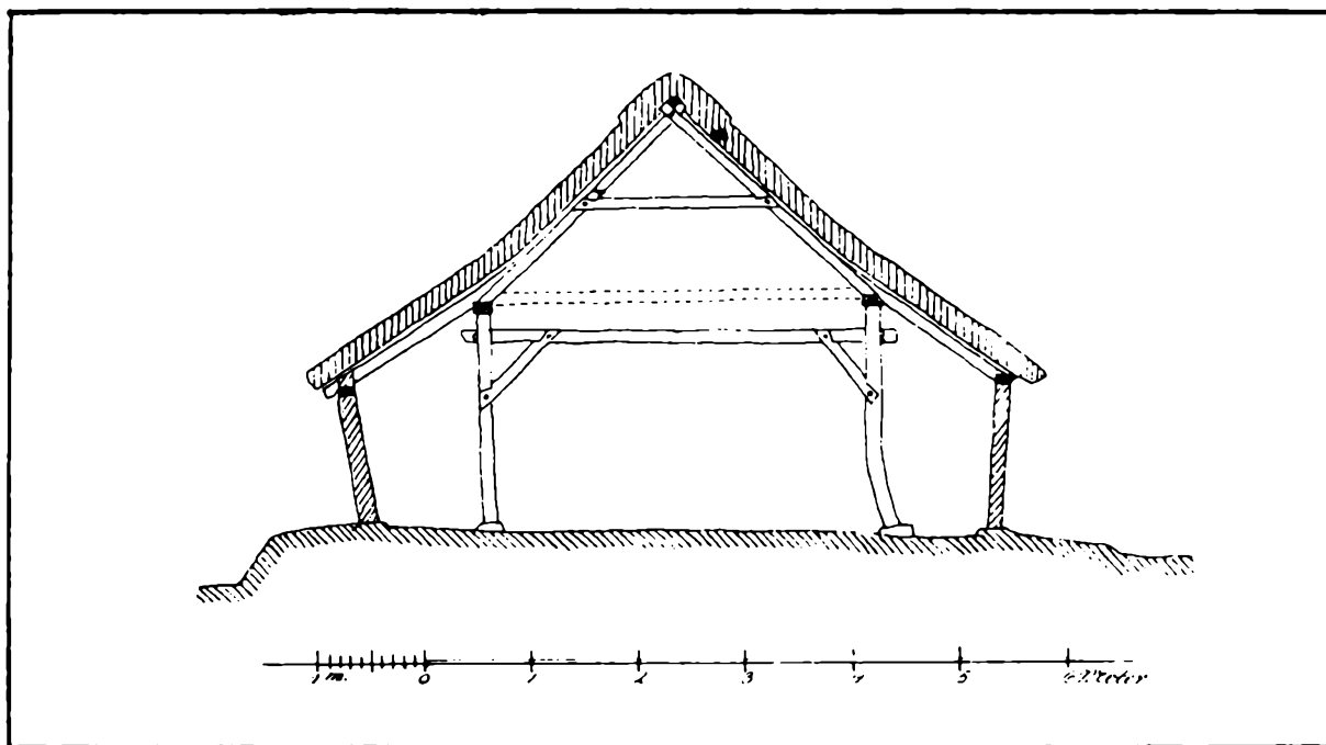
Fig. 1. Tværsnit af et hus fra Agger by og sogn
