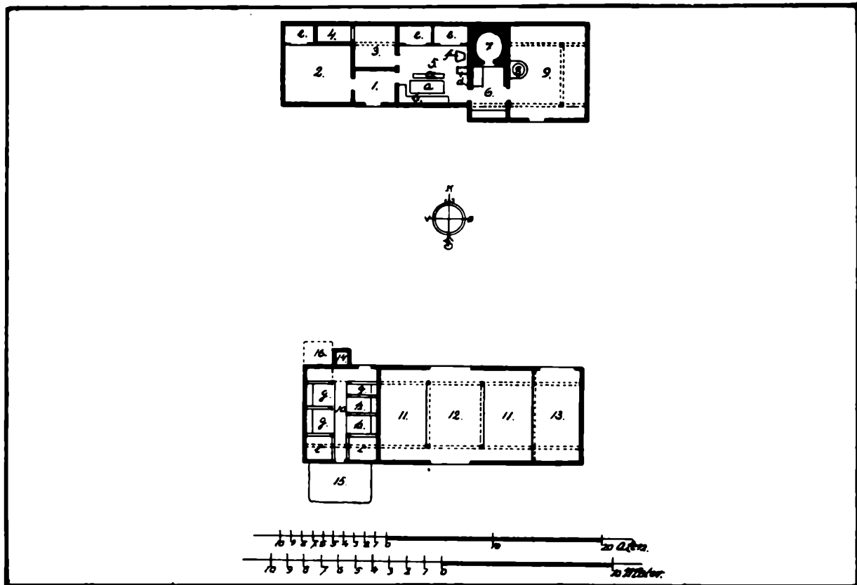
Fig. 6. Grundplan af en gård fra Hjardemaal Klit. 1) Forstue. 2) Vesterstue (storstue). 3) Ølkammer (spisekammer). 4) Saltekammer. 5) Dagligstue. 6) Frammers (køkken). 7) Bageovn. 8) Bryggerkedel (gruekedel). 9) Yderframmers (bryggers) og Tørvehus (ildingshus. 10) Stald. 11) Gulve. 12) Kørelo (også kaldet agegulv). 13) Vognport. 14) Kjeld (brønd). 15) Mødding. 16) Høsehus (senere tilbygget). a) Bord. b) Bænk. c) Skammel. d) Bilægger. e. Senge. f) Armstol. g) Ko- og kalvebåse. h) Hestebåse. i) Grisebøgle.
