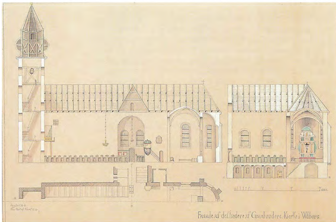
Snit gennem Gråbrødre Kirke tegnet af Chr. Gullev i 1889 længe efter kirkens nedrivning. Tegningen viser den i 1657 tilbyggede »Korskirke«, med underliggende gravkrypt og et kig mod alteret. Det blev solgt til Vorde kirke på auktion i 1813.
