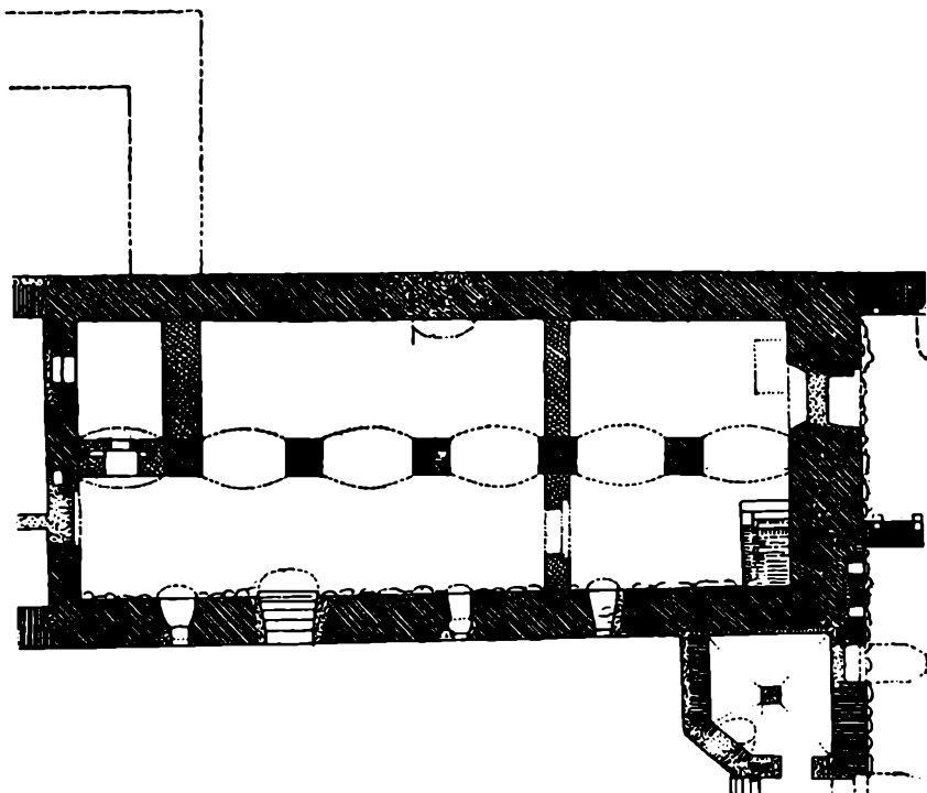
Fig. 8. Kælderplan i Nordfløjen. 1:200 (eft. Ældre n. Architektur VIII).
