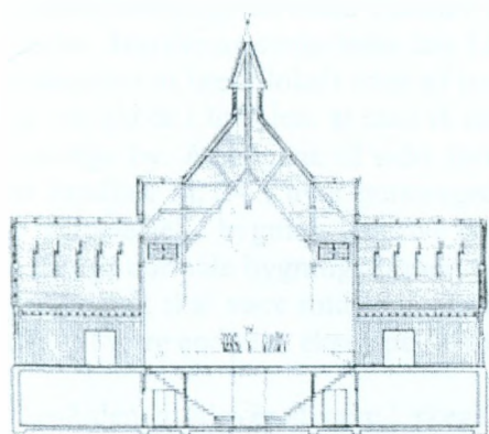
Tværssnit
