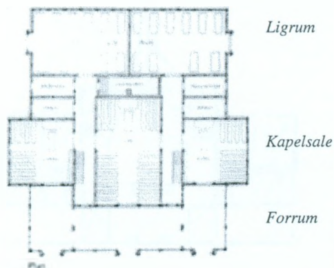
Plan af Østre Kapel i oprindelig udformning fra 1903 Forrummet vender ud mod Frederiksborgvej.
