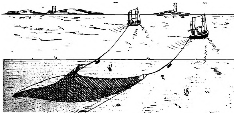
Fig. 3. Vingetrawlen adskiller sig i det væsentligste ikke meget fra den ældre trawl bortset fra, at armene af net er fjernet og forgarnet forsynet med 2 eller 3 vinger (snipper) i hver side (på tegningen 2), hvortil slæbelinerne fastgøres.
