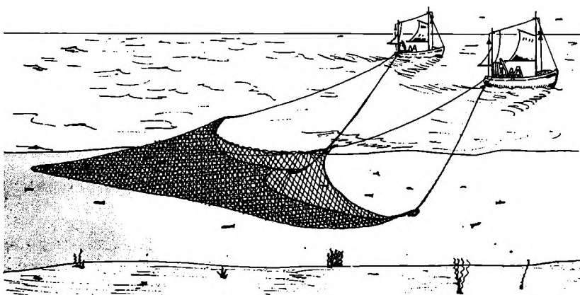
Fig. 4. Flydetrawl.
