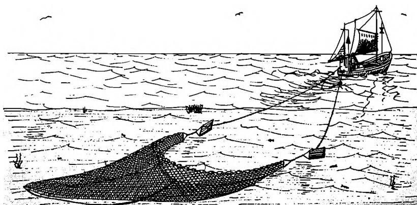
Fig. 2 viser den ældste form for fisketrawl (armtrawl), bestående af pose, forgarn, under- og overlig med henholdsvis vægte og opdriftsmidler anbragte for at holde trawlen åben under slæbning over havbunden. Fortil er nettet skåret til som arme, hvortil linerne mellem trawl og skovle til spiling er fæstnet. Redskabet kaldtes i daglig tale for »armtrawl«. Det anvendes ikke længere.
