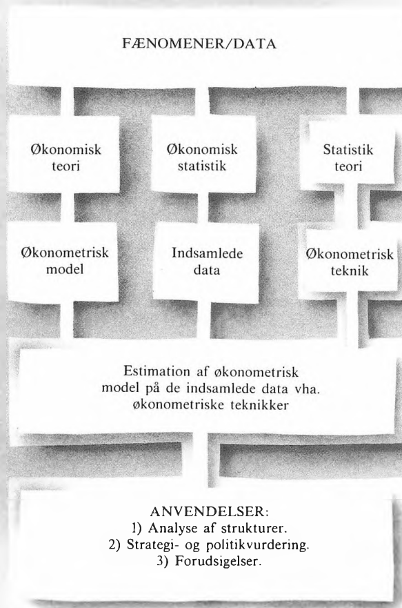
Figur 1. Økonometrisk proces.
