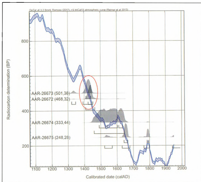
AMS-laboratoriets kulstof14-kurve. De to øverste prøver stammer fra Gl. Skivehus.
