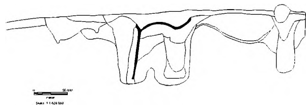
Fig. 8: Snittet tværs gennem højen afsløre, at de to grøfter ikke kan have været samtidige da det tydeligt ses hvordan kammerkonstruktionen (her fremhævet med sort) overlejrer det ene grøftforløb. Skitse: Museum Salling Arkæologi
