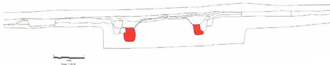
Fig. 4: Tværnit gennem højtomten. Grøftforløbet ses som to nedgravninger. De nederste opfyldningslag er markeret med rødt. Foto: Museum Salling Arkæologi
