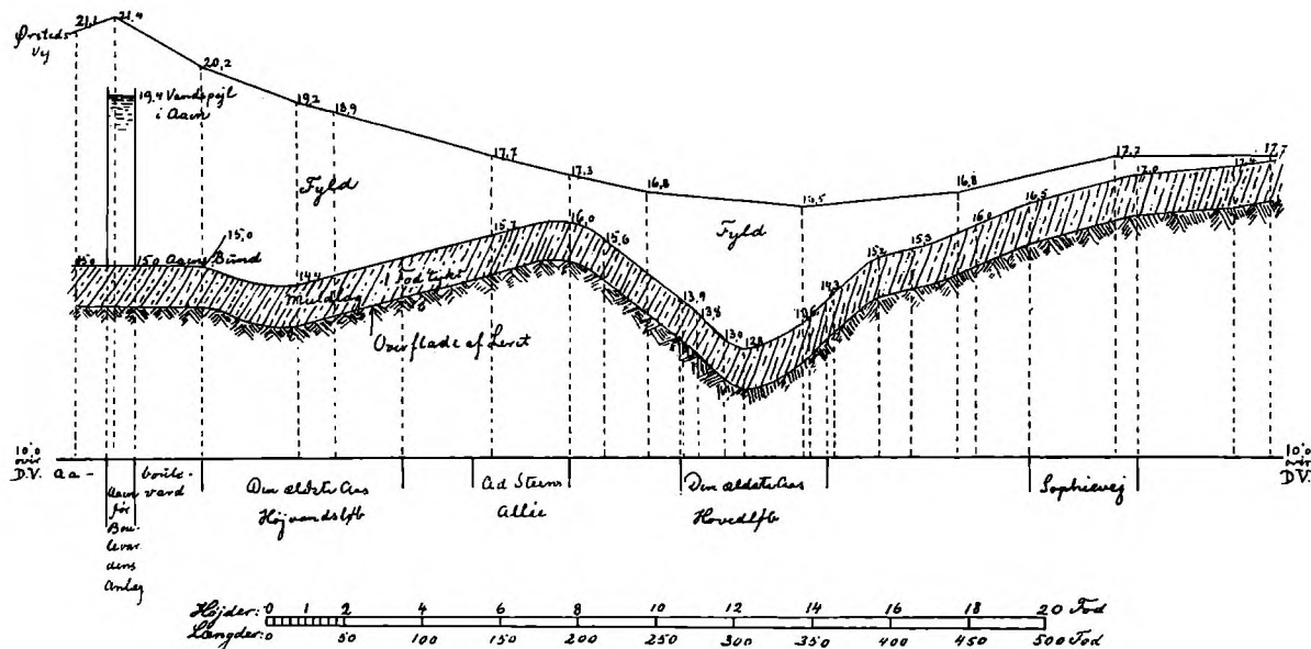
Fig. 3. Profil gennem H. C. Ørsted's Vejs østlige Fortov fra Aaboulevard til Nordbanen, visende Beliggenheden af den ældste Ladegaardsaa's Hovedløb og Højvandsløb, samt vor Tids Ladegaardsaa.
