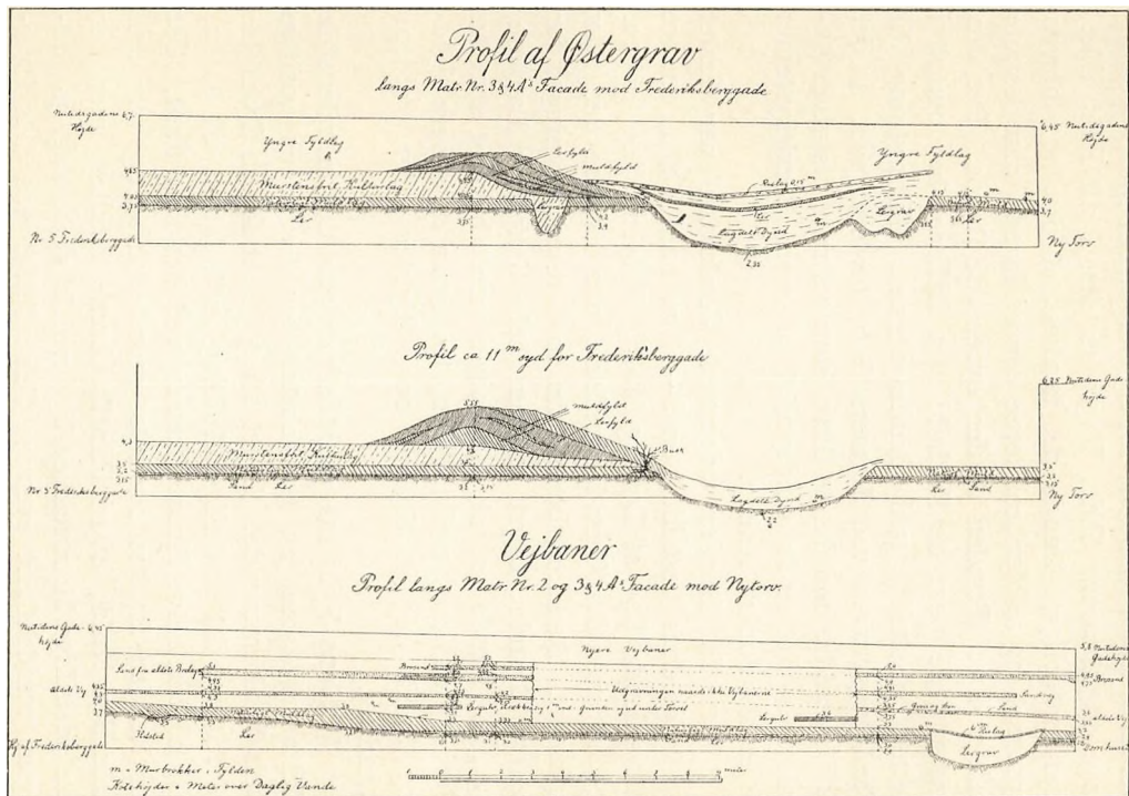
Fig. 3. Profiler af Østergrav og af Vejbaner langs Nytorv.
