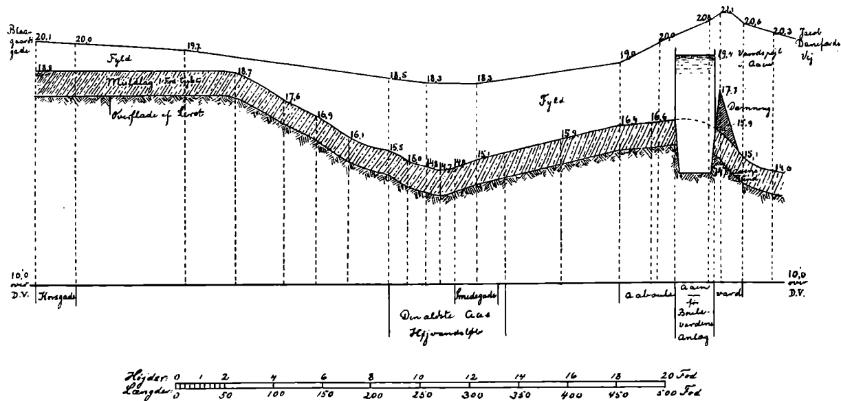
Fig. 4. Profil gennem Blaagaardsgades Vestside og Aaboulevarden fra Korsgade til Jakob Dannefærds Vejs Vestside visende Beliggenheden af den ældste Ladegaardsaas Højvandsløb med hosliggende Dæmning samt vor Tids Ladegaardsaa.
