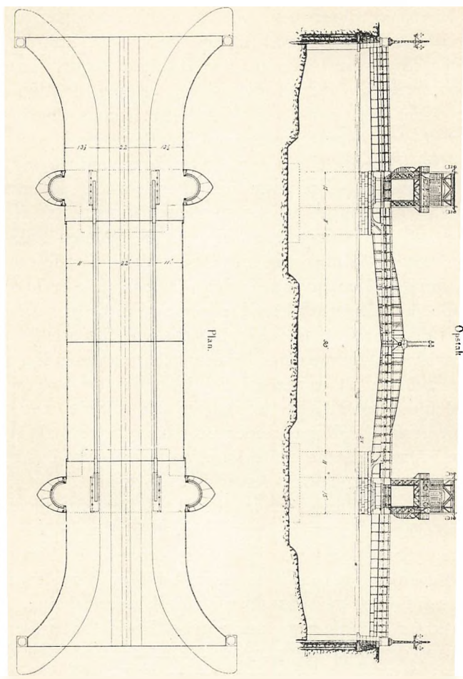
Opstalt og Plan af den nuværende Knippelsbro. Efter Tegning af Forfatteren.
