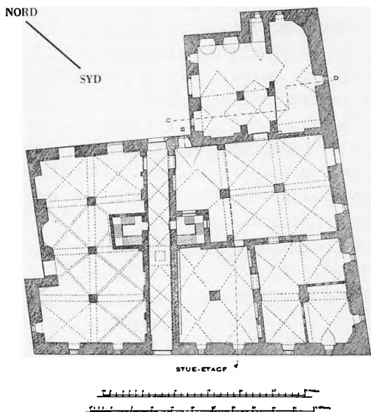
Plan af Christian IV's Bryghus. Fra Ældre nordisk Architectur, V. Saml., 4. R. — Maal 1:800.
