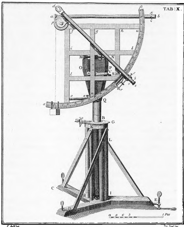
Fig. 4. Den Ahlske Kvadrant. Hoveddelene ses endnu i den astr. Samling paa Rundetaarn.
