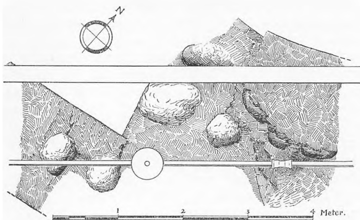
Fig. 2. Detailplan af Fundamenternes søndre Del.
