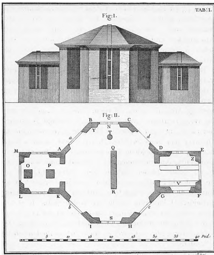
Fig. 3. Bugges Observatorium. Tegning og Grundplan. Murkvadranten stod ved Q R. Meridiankredsens Søjler er O og P.
