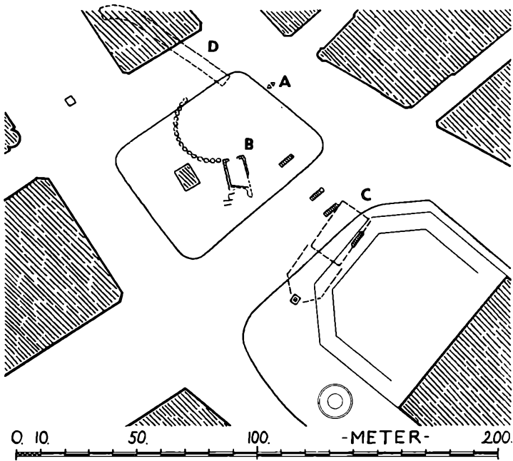
Fig. 1. Plan af Raadhuspladsen. A. Murværk af den ældste Vesterport. B. Vesterports Fundamenter 1931 og 1865. C. Den yngste Vesterport. D. Walckendorffs Hvælving.
