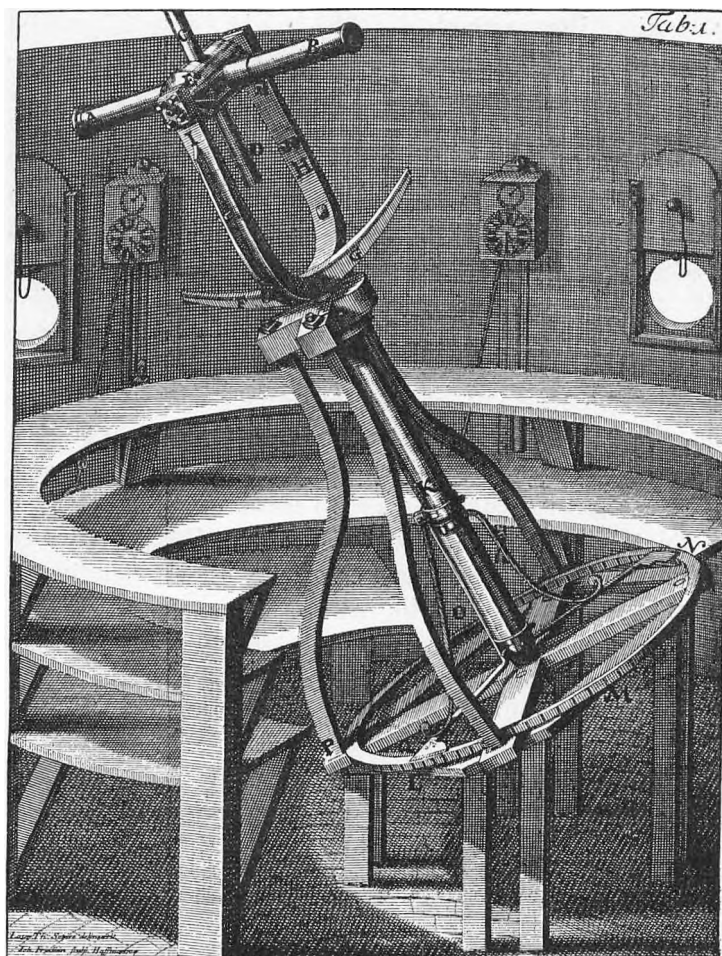
Fig. 1. Ole Rømers Ækvatoraal.
