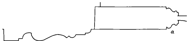
En Barok tofyldings Enkeltdør, Vognmagergade 33, opf. omkr. 1740. Profil a hyppigt i Rokoko.
