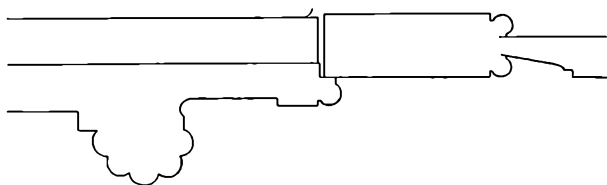
En tofyldings Døbbeltdør i Louis Seize-tidlig Klassicisme, Konge værelset i Vestindisk Tækkhus, af Harsdorff 1780-81.
