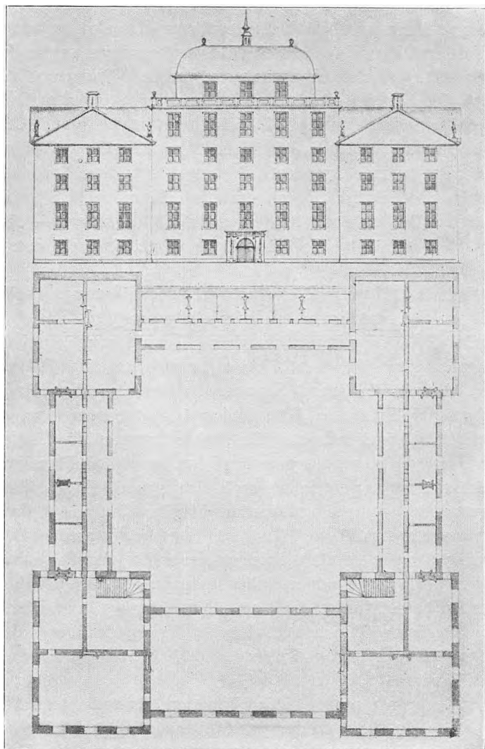
Façade og Grundrids af det paatænkte Slot i Kastelet. „Før og Nu“.
