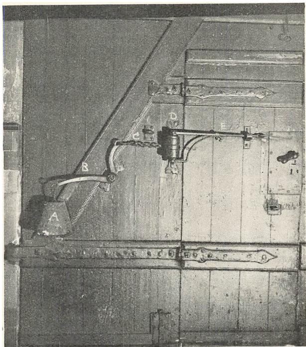
Dørlukker fra Nyhavn 22.
