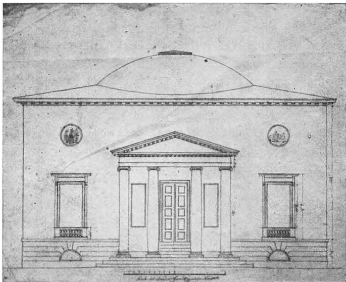
Elbchaussee 157. Facade. Originaltegning af C. F. Hansen. Kunstakademiet. Efter „Samleren“.
