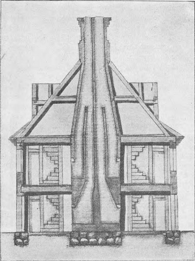
Tværsnit gennem en Dobbeltbarakke. Se S. 211.
