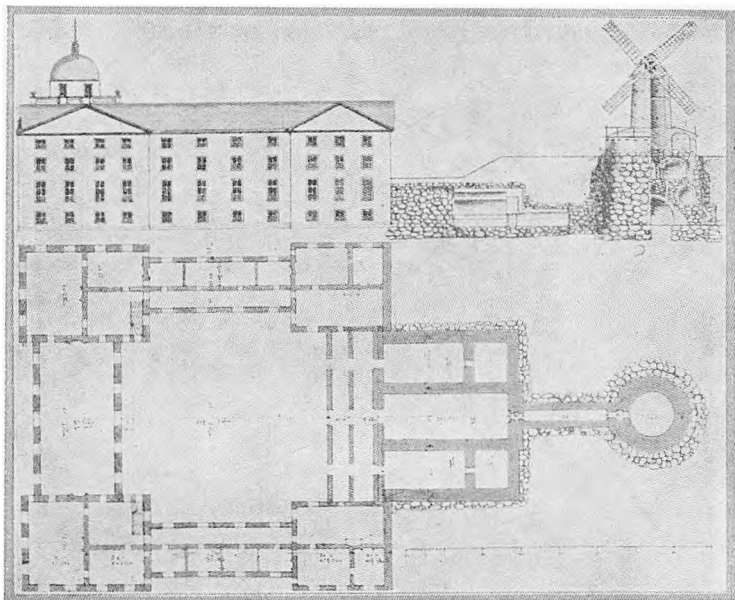
Nordre Sidefaçade og Grundrids af det projekterede Slot i Kastelet.
