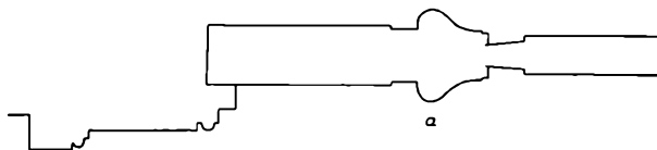
Træ senklassicistisk, femfyldings Enkeltdør, Stormgade 27, sandsynligvis efter Brand 1866. Profil a paa indvendige Døre tilhører Tiden omkr. 1860.
