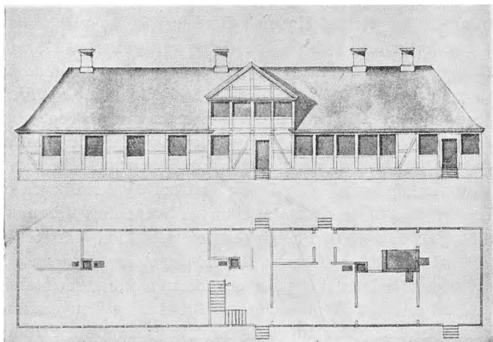
Fig. 2. Tegning til et nyt Gartnerhus paa Frederiksdal efter Generalbygmester E. D. Häussers Forslag 1741.
