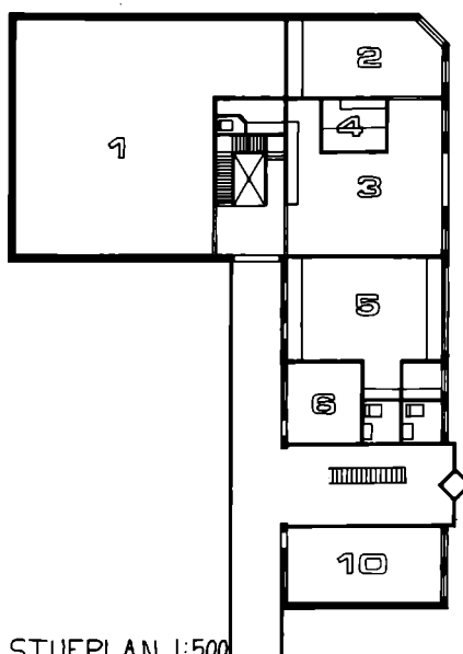
STUEPLAN 1:500
