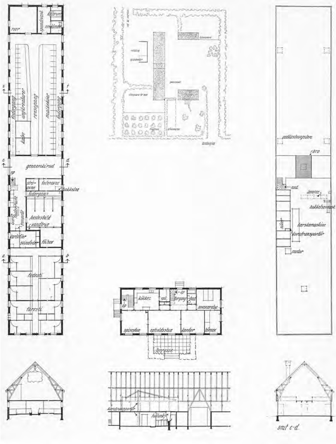
Arkitekt Niels Daugbjerg Bygninger til et Landbrug med ca. 20 Malkekeer. Maal 1 : 400
