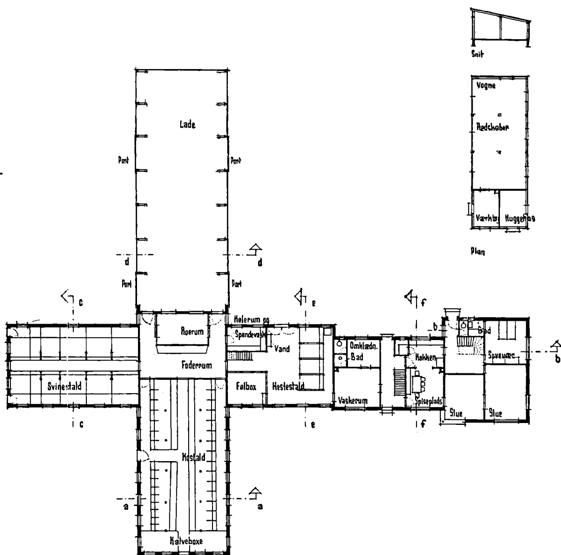
Arkitekterne Otto Jønsen og Kjeld Klitgaard Andersen, Bygninger til et Landbrug med ca. 20 Malkekøer. Mål 1:400.
