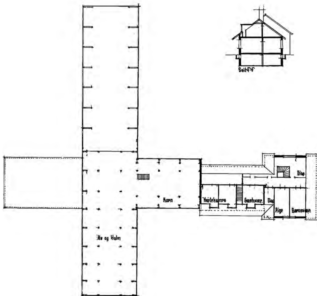
Arkitekterne Otto Jensen og Kjeld Klitgaard Andersen, Bygninger til et Landbrug med ca. 20 Malkekøer. Mål 1:400
