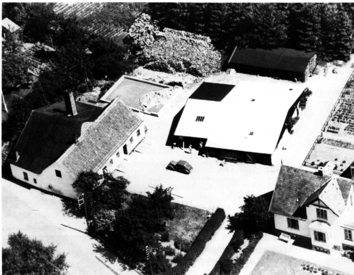
Lillerød Lervarefabrik i slutningen af 1940'erne. Bemærk det store brændelager og æltébassin. Det gamle pottemageri brændte i 1952, men man fortsatte produktionen i lagerbygningen i midten.
