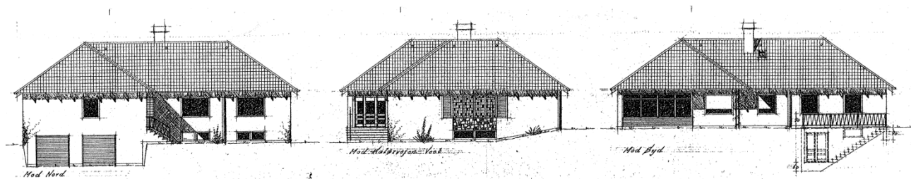
Arkitektens facadetegninger
