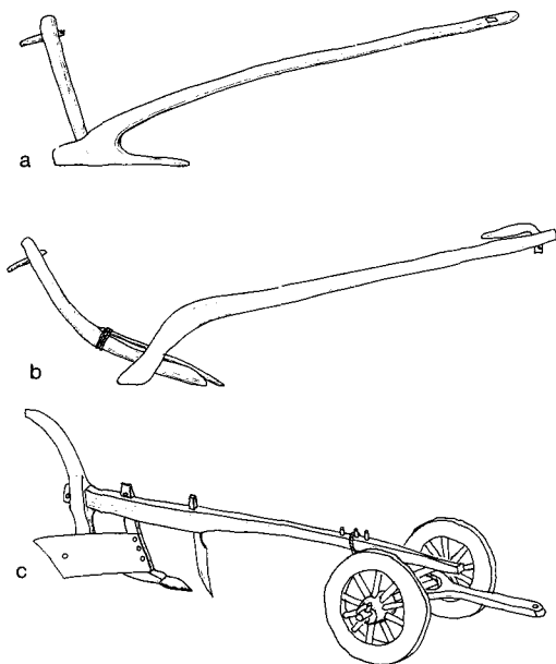
Fig. 2. Oldtidens plovtyper. a: krogard (3500 f.Kr.-800 e.Kr.), b: bueard (ca. 1500 f.Kr.-1000 e.Kr.), c: hjulplov fra vikingetiden med muldfjæl af jern.
