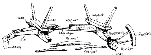
Fig. 5. Træetøj til en stiv arbejdsvogn med jernaksler. Kilde 1.
