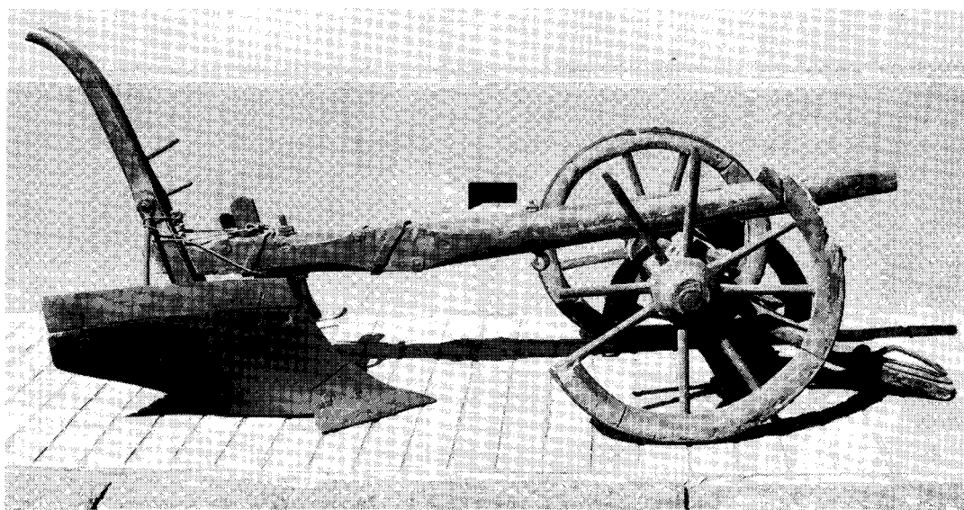
Fig. 9. Hjulplow med smedet plovlegeme og støbt muldfjæl, mærket »O. Strand«. På åsen kan man se, at ploven kunne bruges både som hjulplov og som svingplow med det bornholmske træktøj »stallekiste« sat i det forreste hul i åsen og trækkæden anbragt i krogen under åsen. Altså en slags overgangsform. Muldfjælen er forhøjet med et brædt. Ploven stammer fra Nexø. Foto N.M. 1957.
