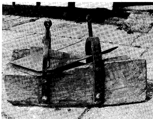
Fig. 8. Træblok med skruevinger, hvori en smedet stålmuldfjæl kan spændes fast under formningen eller under hærdeningen. Blokken stammer fra smed Malmqvist i Rø, men kommer tidligere fra en smed i Rutsker. Foto BM.
