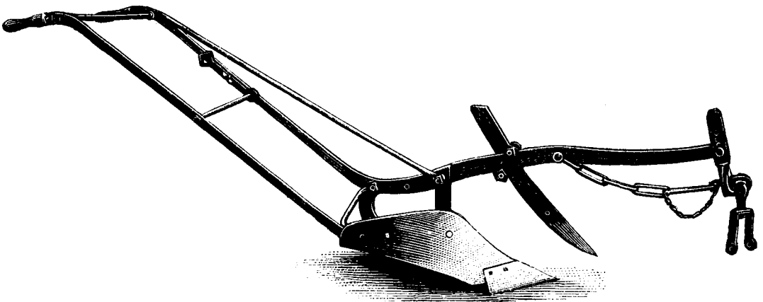
Fig. 10. Bornholmsk »smedeplov«, der deltog i plovprøven på Birkholm ved Herlev i 1898. Desværre var den tungest at trække og brugte hele 89% mere trækraft end den letteste plov. Fra E. Jørgensen: De danske redskabs- og maskinprøver 1902.
