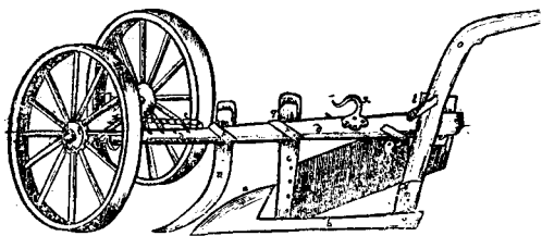
Fig. 2. Sogneedegn Samuel Hertel i Vestermarie konstruerede i 1760'erne en hjulplov, der blev omtalt og afbilledet i Kjøbenhavns Adresse-Cont. Efterretninger no 54, 1763. Det væsentlige er, at åsen hænger under hjulakslen, og slåen c, plovhovedet b samt en del af stjerten m var af jern. Dette skulle give en lettere gang og mindre gnidningsmodstand, så man sparede trækraft. Kgl. Bibl.
