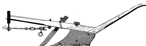
Winstrup's Plov, set fra Landsiden.
