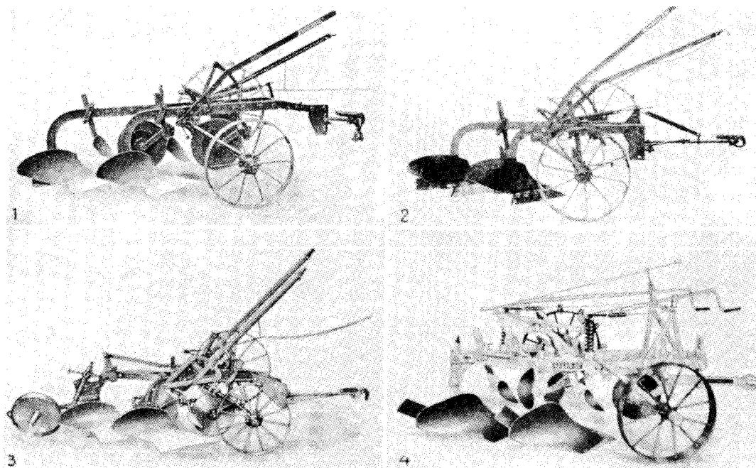
Fig. 12. Fire forskellige bugserede traktorpløve: 1. Fraugde. 2. Sanderum. 3. »Little Genius (I.C.H.)«. 4. Sesam (Överum). Fra H. Rosenstans Schacht. Maskinbog. 1941.
