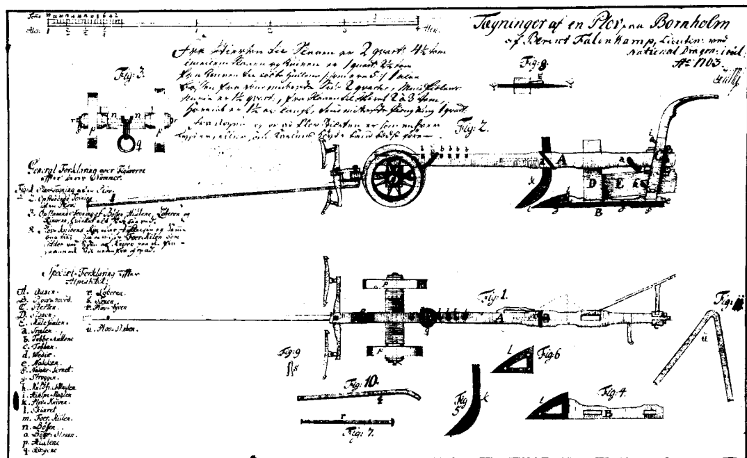
Fig. 1. Tegning af bornholmsk hjulplov udført af løjtnant Berent Falenkamp i 1763, til Urnes agerdykningsbeskrivelse. Der hersker tvivl om denne tegning er en rentegning af Urnes tegning, eller det er en selvstændig tegning. Kgl. Bibl. Thott 1416,4°. På tegningen står følgende:
