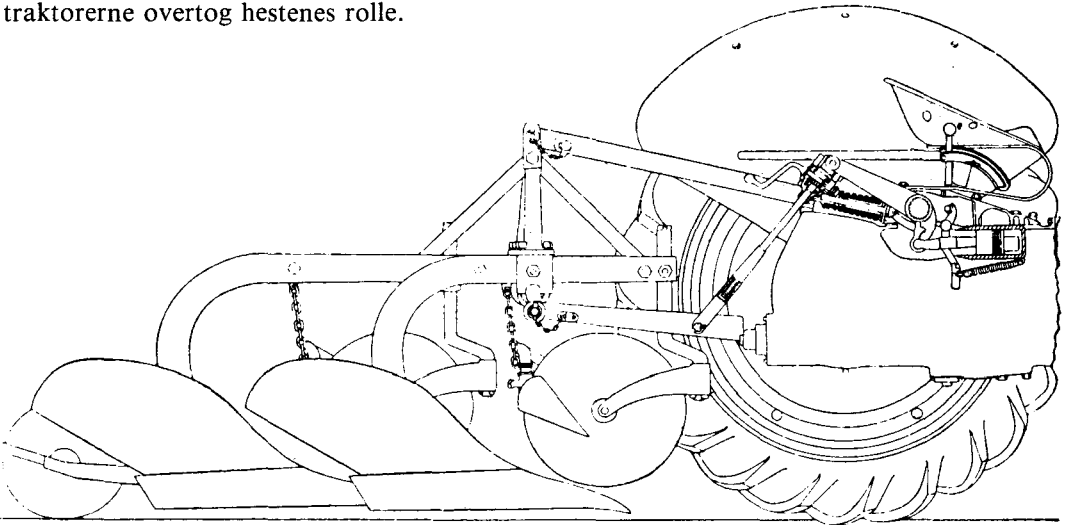
Fig. 14. Tegning af traktor med bærbar plov ophængt i »trepunktsophæng«, der hæves og sænkes hydraulisk, Ferguson, fra Maskinbog for landmænd 1951.
