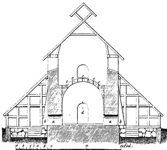
Snit og grundplan af en hvælvet kammerovn med plads til ca. 50.000 sten. Dimensionerne er 7,5 \times 3,8 \times 3,8 m. a. Indfyringshuller, b. Afstivere, c. Røghuller, og d. Indtrilningsdør.
