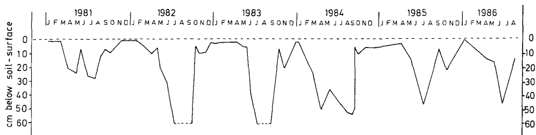
Fig. 17. Kurve visende variationen af højden af den fri vandoverflade i forhold til jordoverfladen (stiplet linie) i en m.el.m. afløbsløs lavning i Borrelyngen afd. 690.
