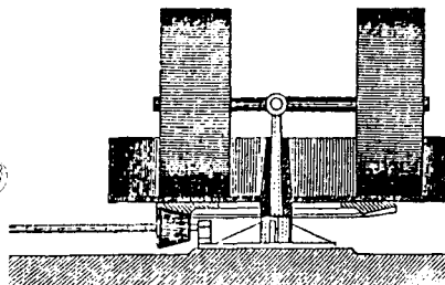
T.v. englænderen I. Hunts murstensmaskine med valser, patenteret i 1843. For at trække leret ned var valserne omgivet af et endeløst klæde. Forneden overskæres lerstrengen i passende stykker, og de enkelte sten transporteres bort fra maskinen på en kæde uden ende. T.h. en kollergang til lerbearbejdning. Den viste konstruktion er med roterende skål.
