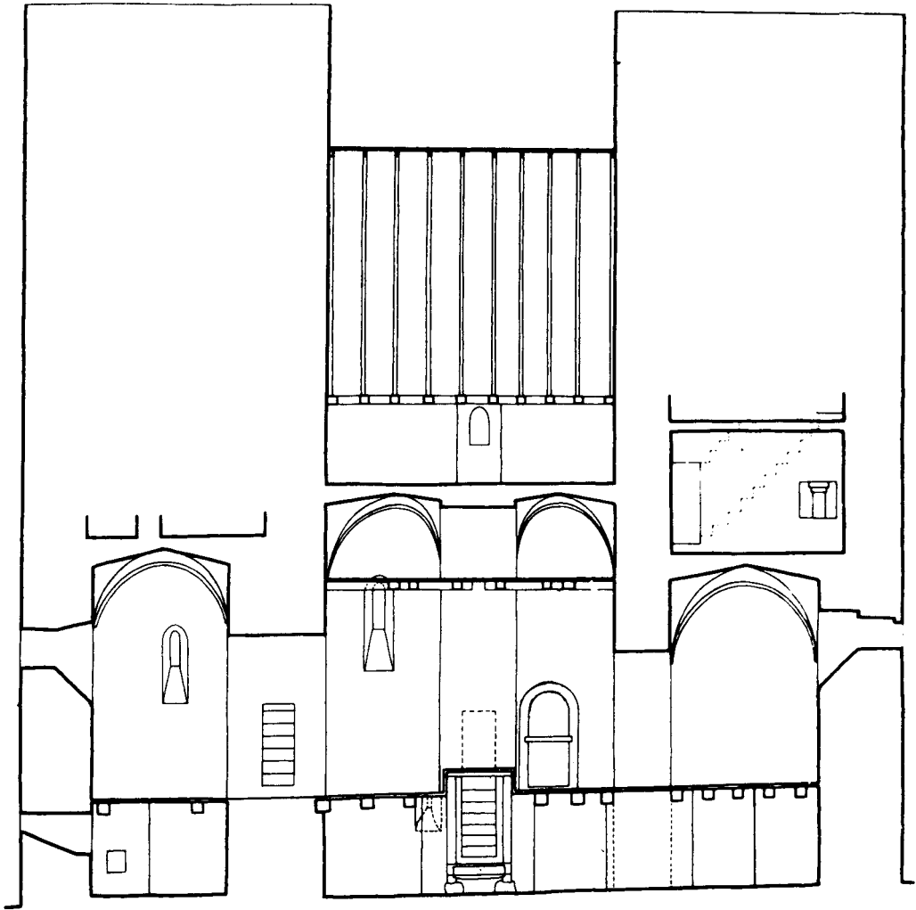
Fig. 3. Halltorps kirke. Rekonstrueret længdesnit, set mod syd (Halltorp II). Efter kyrkorna i Stenäs och Haltorp (se litteraturliste).
