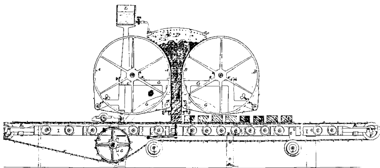
T.v. englænderen I. Hunts murstensmaskine med valser, patenteret i 1843. For at trække leret ned var valserne omgivet af et endeløst klæde. Forneden overskæres lerstrengen i passende stykker, og de enkelte sten transporteres bort fra maskinen på en kæde uden ende. T.h. en kollergang til lerbearbejdning. Den viste konstruktion er med roterende skål.
