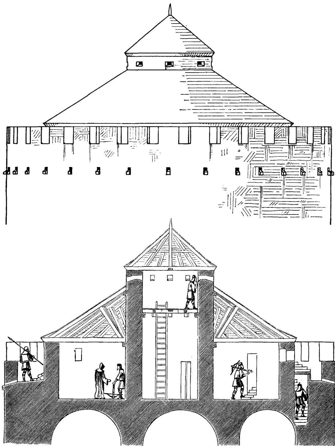
Professor F. Laskes rekonstruktion af Østerlars Kirke.
