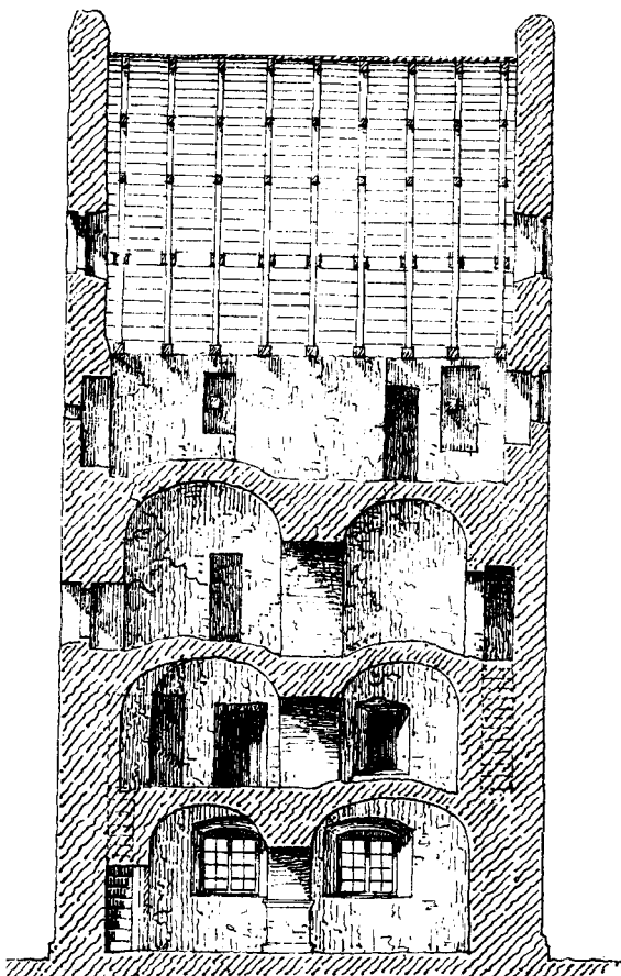
Fig. 4. Ibs kirkes vesttårn i tværsnit set fra øst. Skala ca. 1:200. Tegning i Holm 1878.
