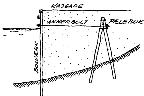
Skitse til det, Thorsen kalder »bukkede pæle«.
