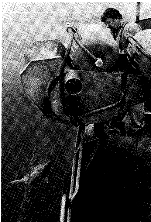
Med selvhaleren, der drives hydraulisk, hives de tunge torskegarn op gennem vandet og indenbords. Hjælpe midlet sparede fiskerne for det hårde indhalingsarbejde og er en af de faktorer, som har været med til at effektivisere fiskeriet betydeligt. R 282 "Jesper" af Årsdale. Foto. P. H. Moustgaard 1985.
