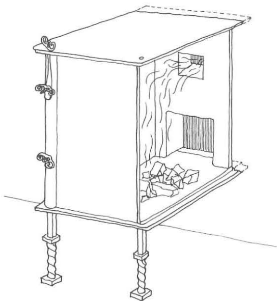
På tegningen, hvor den ene sideplade er »fjernet«, kan man se bilæggerovnens princip. Den er muret ind i en væg med tilslutning til en skorsten med åbent ildsted, hvorfra man fyrer i bilæggeren. Der er to huller, foruden indfyringshullet nederst et røghul. Tegning Niels-Holger Larsen.
