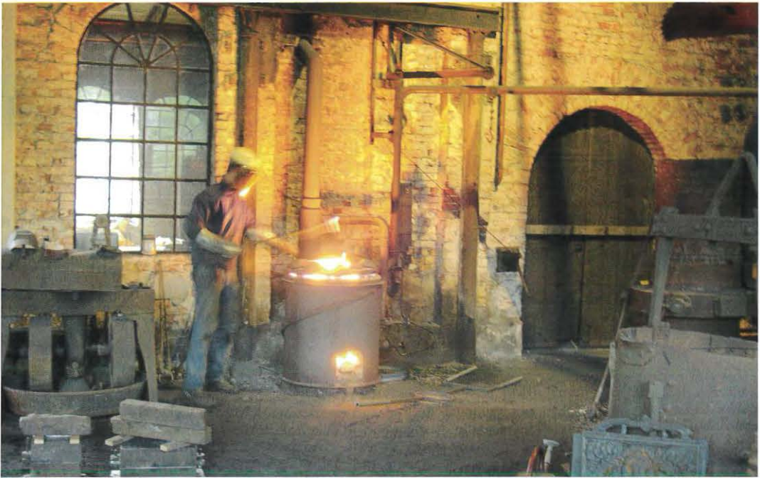
Råjernet smeltes på Ebbamåla Bruk i Blekinge. I højre nederste hjørne ser man en del af en nystøbt dronninge-ovnplade, som endnu ikke er afrenset for støbegrater. Endnu i dag kan man på dette jernværk i Blekinge følge hele støbeprocessen. Ebbamåla, der først blev grundlagt i 1885, er i dag også et »industriminde« og museum, hvor man en gang om ugen i sommerhalvåret demonstrerer den næsten magiske arbejdsproces. Foto Niels-Holger Larsen, 2007.
