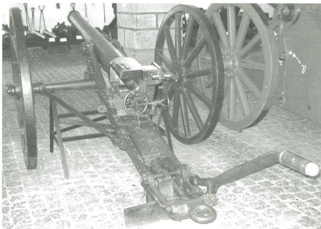
Den Schouboe'ske nødløsning efter tabet af de fire feltkanoner: 75 mm stålskanon L/28 M1894. (Forfatterens foto fra Statens Forsvarshistoriske Museum)
