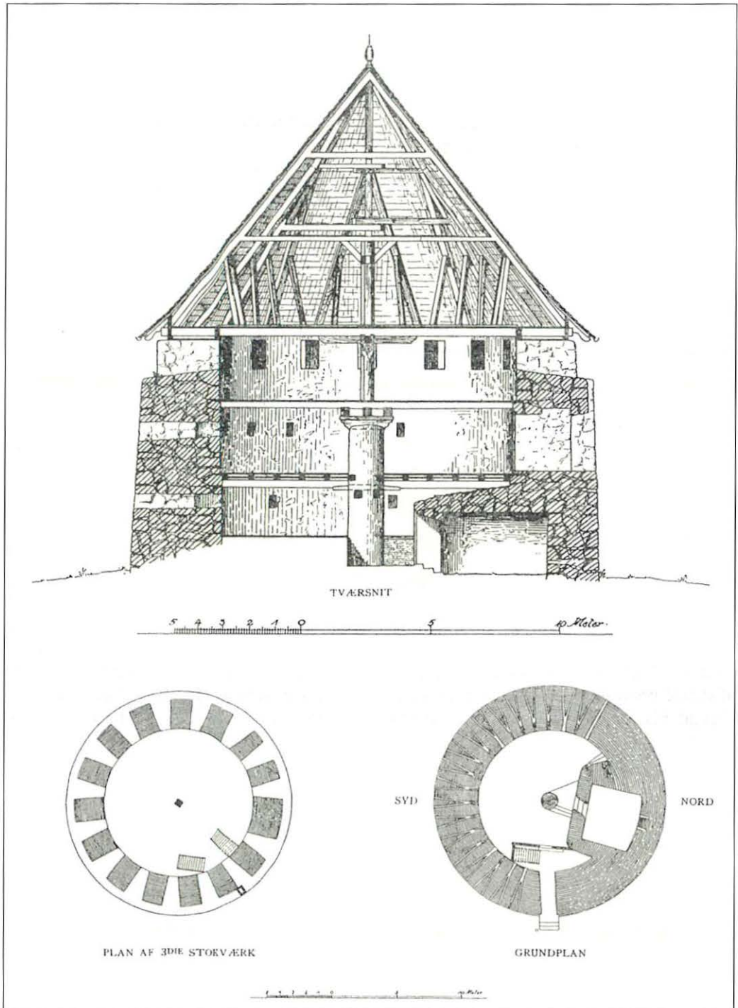
Opmåling af kasteltårnet 1912 (J. Klindt-Jensen: Barokken i Rønne fæstning. Rønne 1952 s.32, fig.19)
