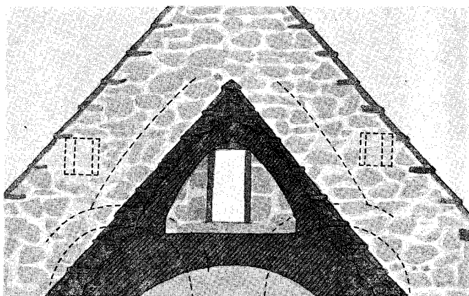
Øster-Marie. Udsnit af Andr. Clemmensens rekonstruktionsskitse vedr. sandstensflagernes anbringelse på taget. Snittet i koret er set ind imod skibets østgavl. Med brudt streg har forf. indtegnet hvælvingsporene på gavlens vestside og de to i teksten omtalte (yngre) lyssprækker. Mål ca. 1 : 100.
