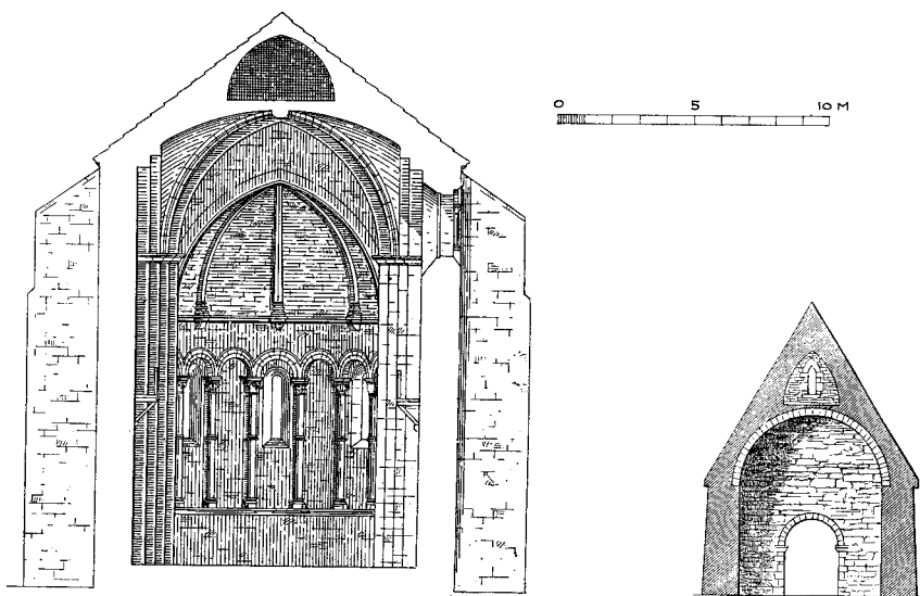
T. v.: Ste Marie au Lac i Le Thor, Frankrig. Slutn. af 12. årh. Snit i skibet set mod koret (efter Debio og Bezold 1887).
