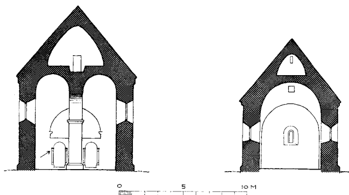
Øster-Marie. Rekonstruerede snit i skib (t.v.) og kor (t.h.) med de oprindelige, massive tagkonstruktioner. Tegn. af forf. efter A. Clemmensen. I snittet til venstre ses ind imod triumfvæggen, hvor forf. har antydnet en muret korsranke, hvis tilstedeværelse er påvist af Smidt og Schultz. Pilen viser den sandsynlige placering af det i artiklen efterlyste søjlefragment. Mål ca. 1 : 300.
