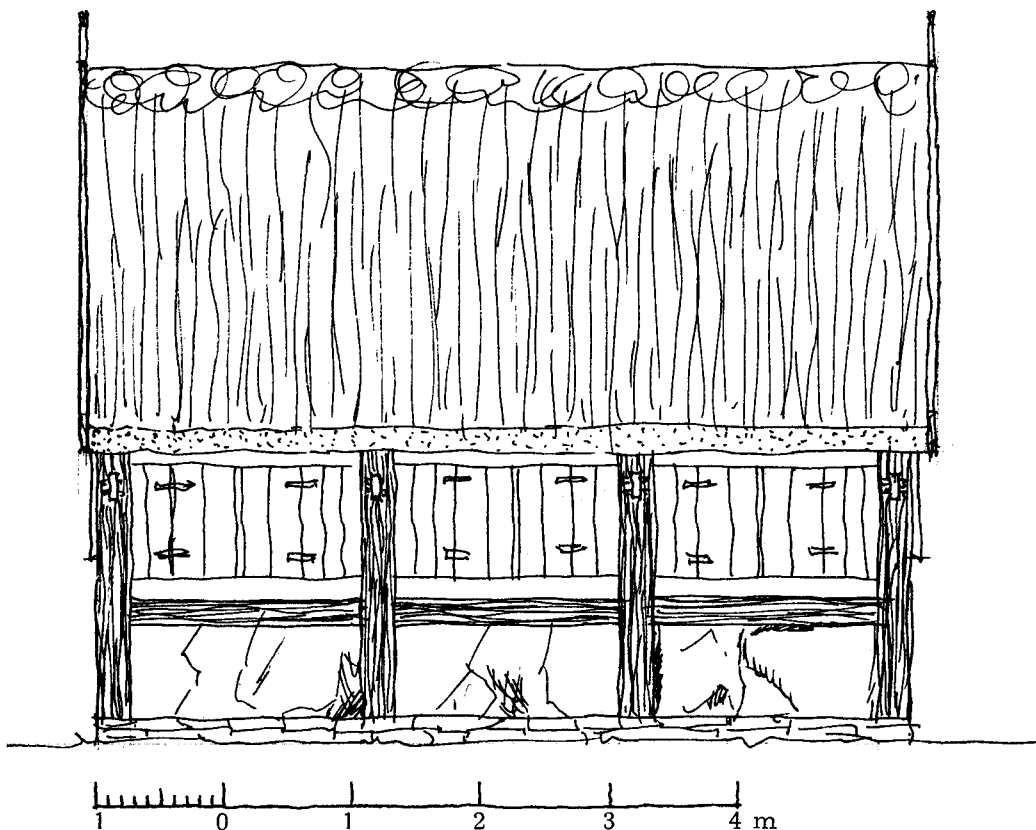
Fig. 9. Rekonstruktion af Klækkehusets langfacade (mod vest).
