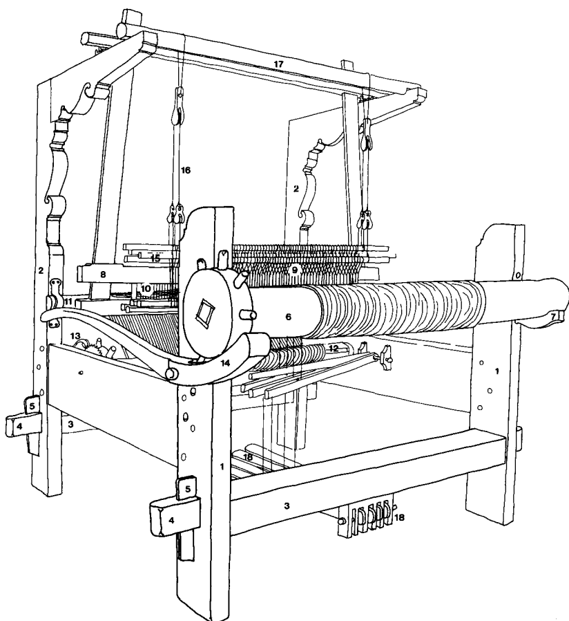
Fig. 5. Tegning af bornholmsk væv med udskårne gavle.
