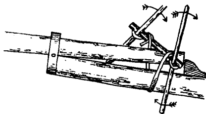
Fig. 257. Spansk Vindse, anvendt til at tvinge en Klyverbom paa Plads.
