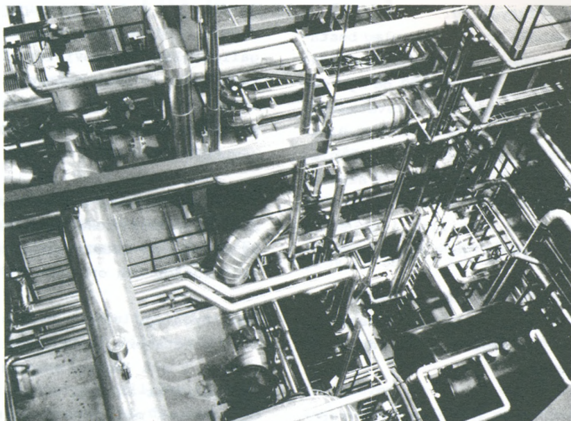
Fjernvarmeladepumpe.
