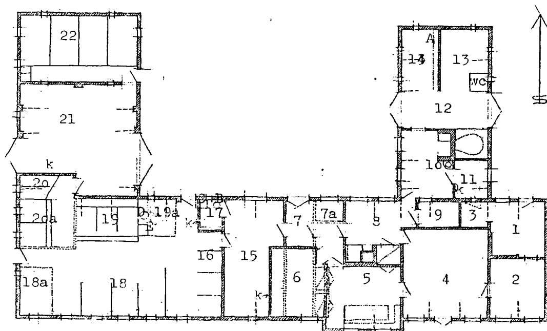
Grundplan af gården Varming Vesterby 25. Opmåling 1947. 1. Tidligere køkken. 2. Tidligere stue. 3. Tidligere brændsels-rum. 4. Storstue eller sal, nogle steder kaldet pissel. 5. Dagligstue, døns. 6. Sovekammer, som tidligere var en del af 7. 7. Forstue eller frangel. 7a. Tidligere spisekammer. 8. Køkken. 9. Pigekammer. 10. Bryggers. 11. Kældere. 12. Lo. 13. Brændsel, tidligere tørvelade. 14. Tidligere fårest. 15. Lo. 16. Heste. 17. Karlekammer. 18. Køer. 19. Kalve. 20. Roer. 20a. Tidligere høgulv. 21. Lade, tidligere hølade. Tidligere var 20, 20a og 21 ét rum. 22. Svin, ny tilbygning.
