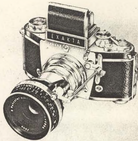
Bild 17 Ihagee „EXAKTA Varex IIa/1961“ mit Bajonettingen und Tuben, Auslöserbrücke und Normalobjektiv mit vollautomatischer Springblende
