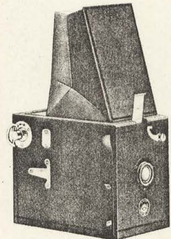
Bild 4 Ihagee „Roll-Paff-Reflex“ 6×6 cm
