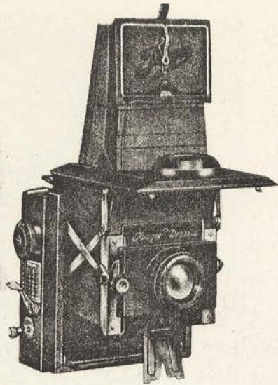
Bild 5 Ihagee „Patent-Klappreflex“ 6,5 x 9, 9 x 9, 9 x 12 und 10 x 15 cm
