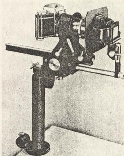
Bild 12 „Ihagee-Vielzweckgerät“ (Reprogerät mit Balgennah-einstellgerät und Diakopiervorsatz)
