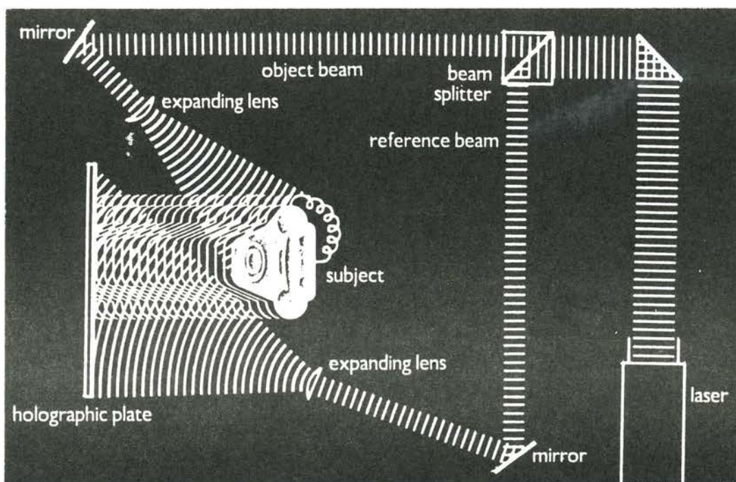
Figur 1 Optagelse af et reflektionshologram
