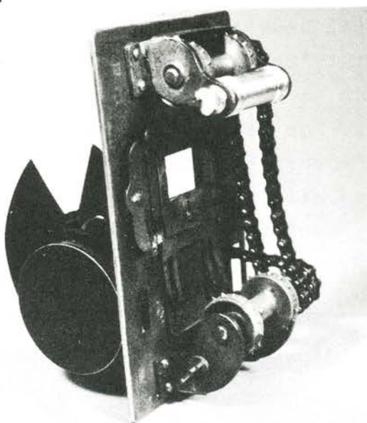
Fremføringsmekanismen med malteserkors.
