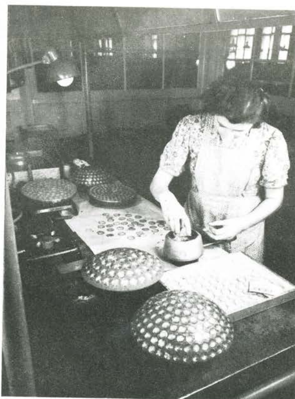
Linser kittes fast i lappetixturer ved hjælp af shellak. Det sker ved 140^{\circ}\text{C} .
