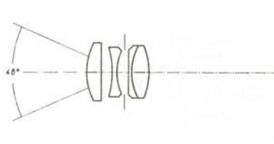
5. Skopar 1:3,5 und 5a. Color-Skopar 1:2,8
