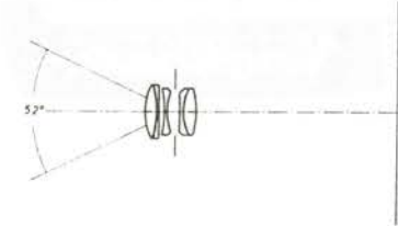
4. Heliar 1:4,5 und 4a. Color-Heliar 1:4,5
