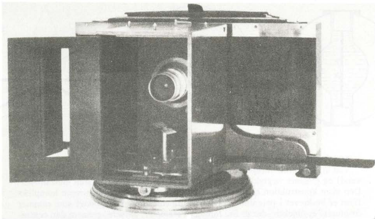
Johnson & Harrison's Phantoscopic kamera. Patenteret den 5. september 1862. Objektiv Grubb-Aplanat. Til 110° billedvinkel på plane kollodiumplader.
