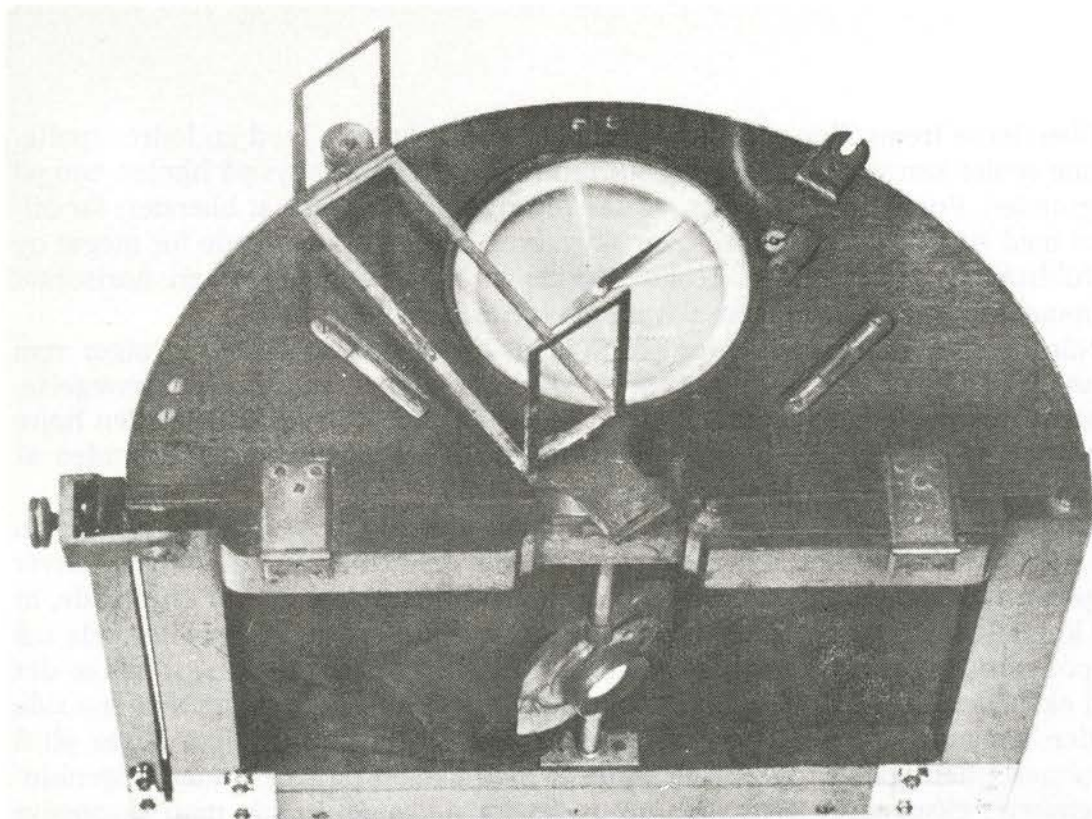
Cylindrographe fremstillet af Moëssard. Patenteret den 17. juni 1889. Objektiv Aplanat 1:8/150 mm.
