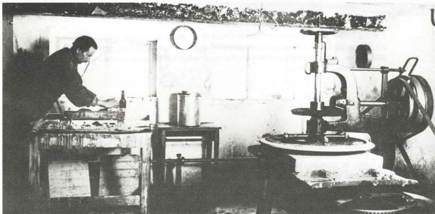
Klichéfremstilling var i 1880'erne en forholdsvis ny teknik. Endnu kunne man kun gengive stregtegninger. En sådan blev fotografisk overført på en præpareret zinkplade. De belyste partier på pladen blev derved gjort syrebestandige, mens pladens øvrige del kunne ætzes. Det færdige resultat var en kliché, hvis motiv stod i svagt relief og derfor kunne trykkes i en bogtrykpresse. Personerne i forgrunden er i færd med at indvalse klichéerne med et syrebestandigt stof, således at tegningens kanter ikke bliver beskadiget af syren. I baggrunden er kemigraferne i færd med at ætse klichéer i store keramikkar. Man anvendte ofte salpetersyre som ætsemiddel.
