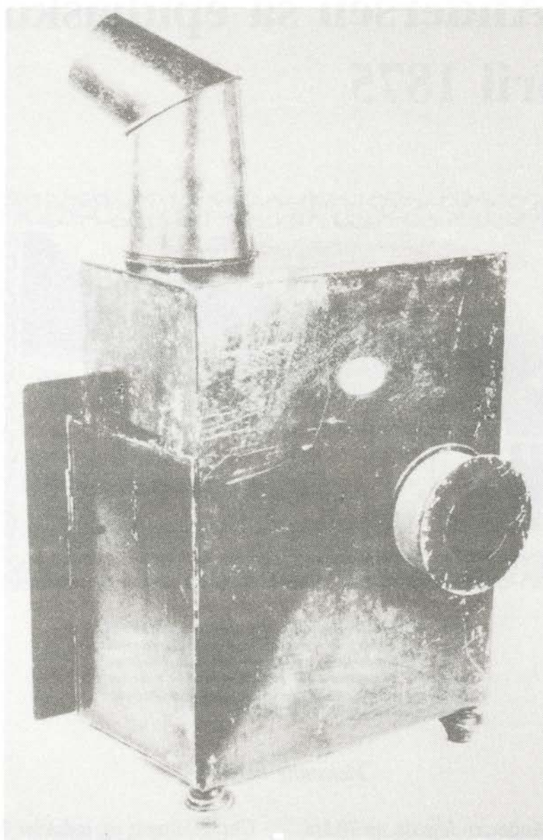
De 14 billeder kan være blevet forevist i et epidiaskop som dette. Epidiaskop ca. 1873-78. Fabrikat C. Eckenrath Berlin. Beregnet til papirbilleder og glasnegativer. Et vippespejl kunne udskiftes med snække/objektiv. Lyskilden var petroleum.
