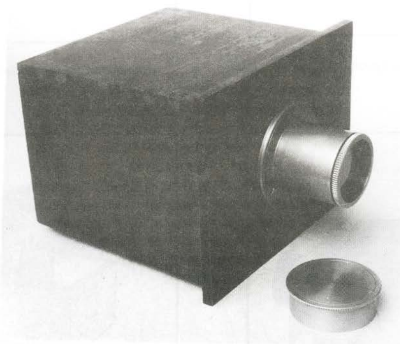
Den indre kasse med linse og dæksel.
