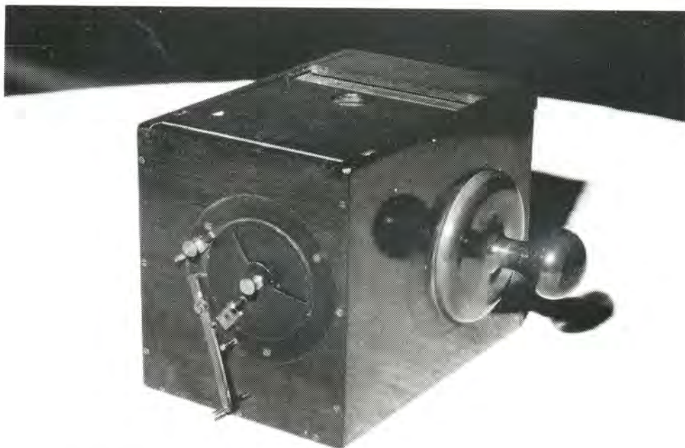
Kameraet set forfra. De 6 stk. (9x12) dobbelt-kassetter tilkobles en sprække på kameraets side. På venstre side er anbragt en knop som håndtag.
