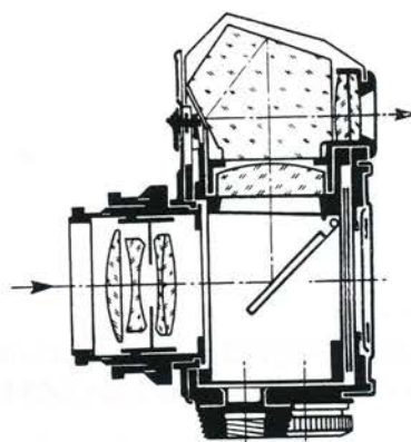
Snit gennem Exakta Varex med prismesøger.
