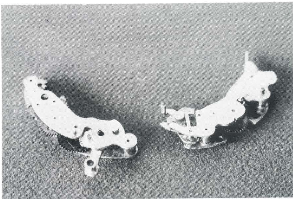
De afmonterede hemværker fra Prontor-lukkeren. De sidder fast med 2 skruer og 1 fjeder.
