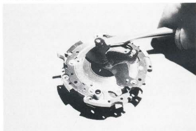
Lukkerbladene lægges på plads.
