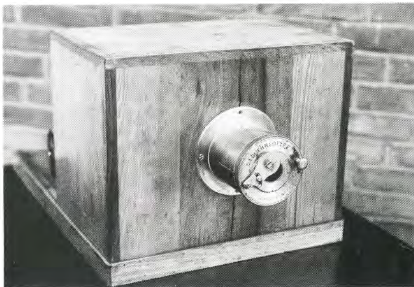
Kameraet til Lerebours daguerreotypi-apparat, som i efteråret 1839 blev anskaffet til den militære højskole. Danmarks Tekniske Museum, Helsingør. Foto: F. Berendt.
