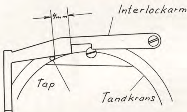
Tandkransens stilling ved indgreb
