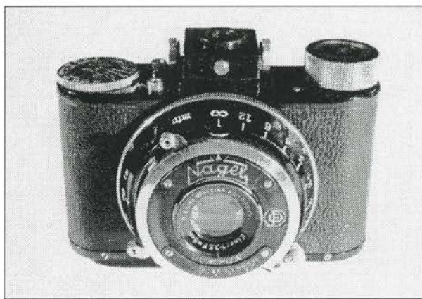
Pupille fra 1930 til 3x4 med Compur og Leitz Elmar. Bemærk dybdeskarpheeds skalaen: Retina'erne blev senere forsynet med samme skala.
