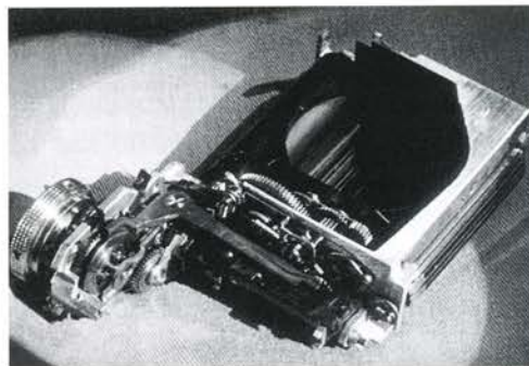
Luk- og optrækmekanismen i Contax II/III. Foto: P. Hennig
