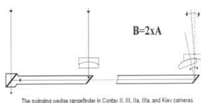
Skematisk gengivelse af afstandsmåleren i Contax II og III med sammenkittet prisme, lang glasbjælke, og svingkile
