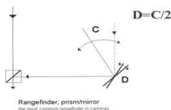
Skematisk gengivelse af Leicaafstandsmåleren med 2 sammenkittede trekantprismer og bevægeligt spejl
