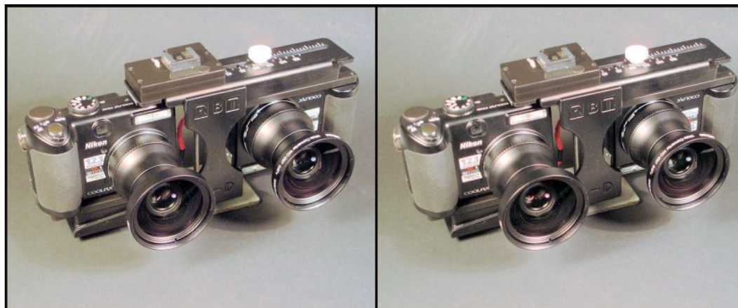
RBT digitalkamera baseret på Nikon coolpix PS100 med 12 megapixel. Kameraet her vist med vidvinkelconverter
