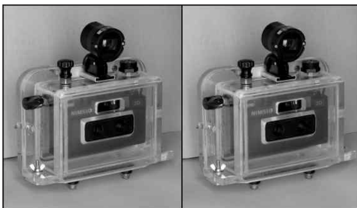
Stereoskopisk undervandskamera med modificeret Nimslo kamera
