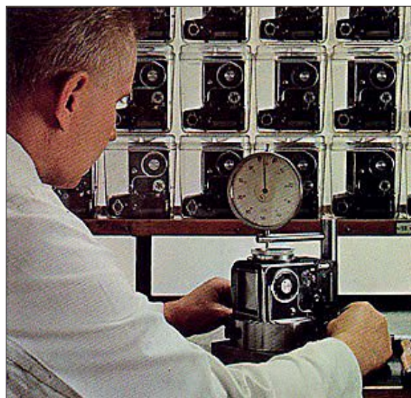
Basismålet kontrolleres på 500 EI
