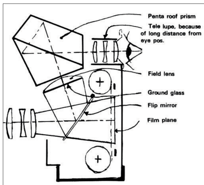
Principskitse af forgængereren, den hemmelige prototype Syntax. Tegnet i 1981 efter erindringen af Zeiss Ikons tidligere konstruktionschef Hubert Nerwin.
